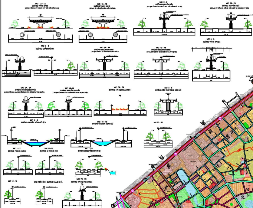
MẶT CẮT NGANG ĐIỂN HÌNH
